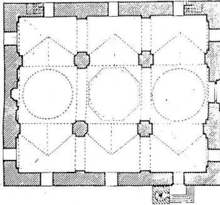
ULUCAMİ PLANI (E. H. Ayverdi'den işlenerek)
